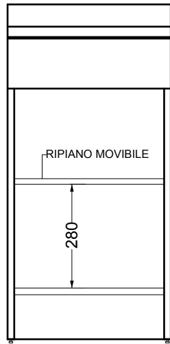
VISTA FRONTALE SENZA PORTE
