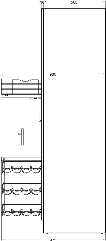
VISTA LATERALE
