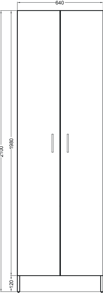
VISTA FRONTALE
