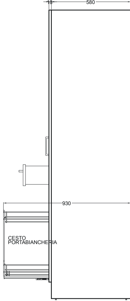
VISTA LATERALE
