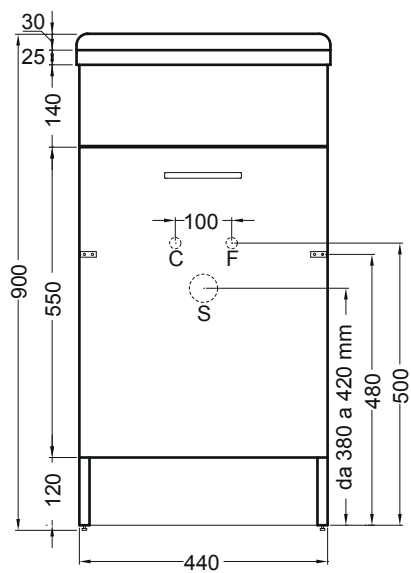
VISTA FRONTALE
