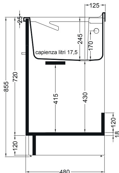
SEZIONE A-A'
