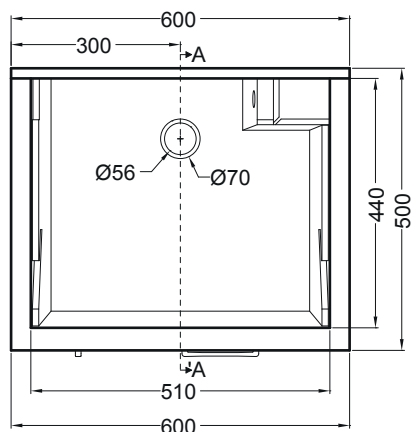
PIANTA
