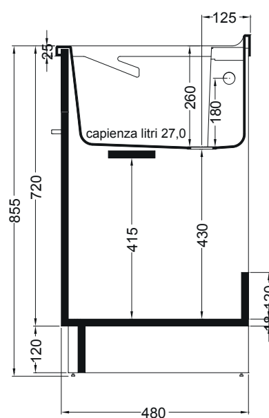
SEZIONE A-A'
